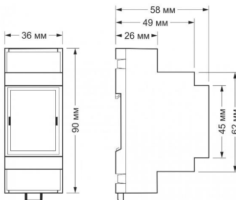
Габаритные размеры SH-DO8.04IS1
