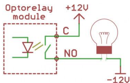
Пример схемы подключения SH-DO8.04IS1
